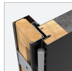
Ościeżnica DUOTHERM 60
