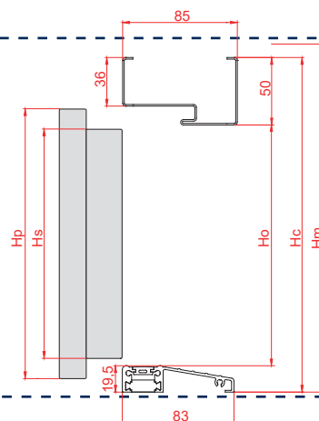
DUOTHERM 75
