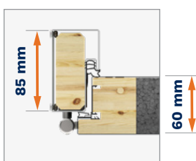
Ościeżnica DUOTHERM 60
