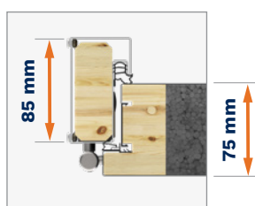
Ościeżnica DUOTHERM 75
