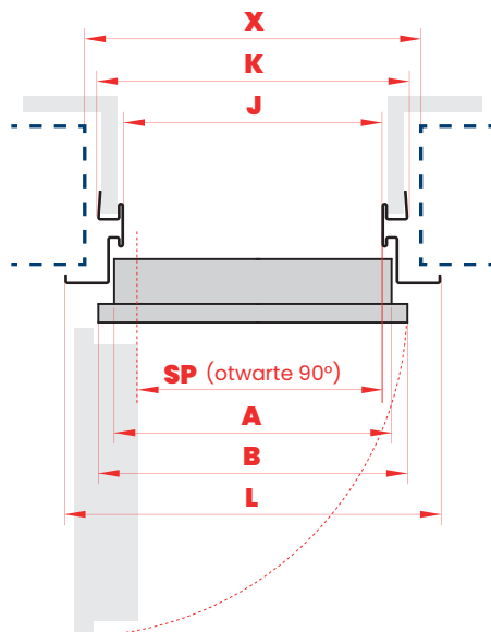
PRZEKRÓJ POZIOMY
