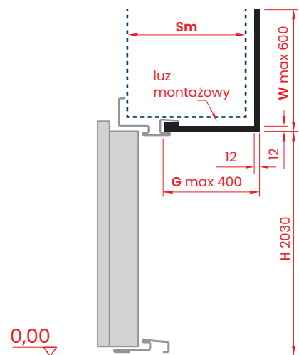
PRZEKRÓJ PIONOWY
