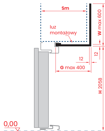
PRZEKRÓJ PIONOWY
